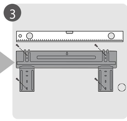
Προσαρτήστε τη βάση τοποθέτησης
