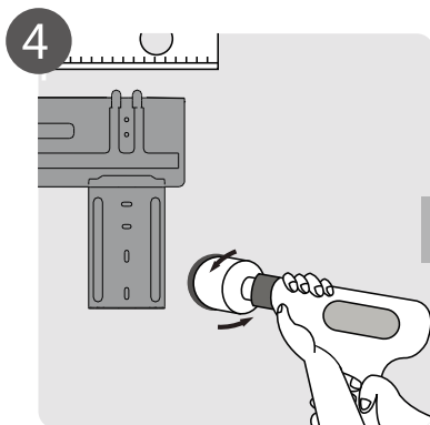
Επιλέξτε τη θέση τοποθέτησης
