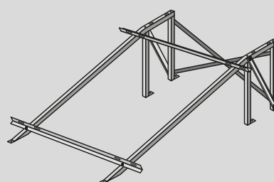
ΒΑΣΗ ΗΛΙΑΚΟΥ Χαμηλού ύψους με 30° κλίση 160-300Lt
